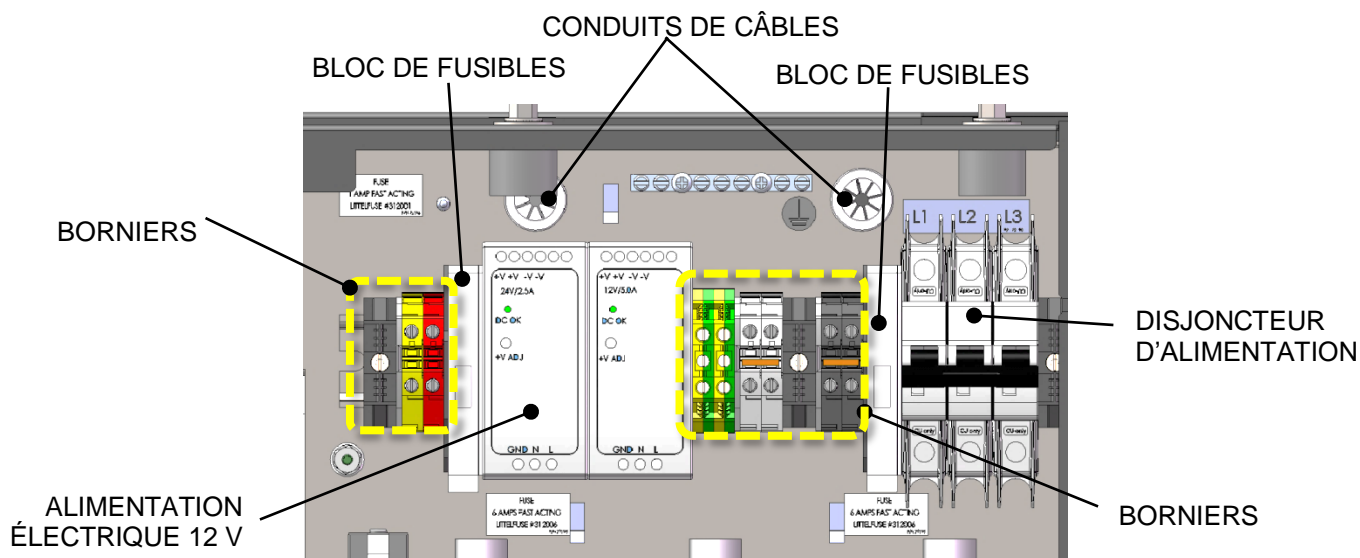
Figure 2-13 : Panneau d'alimentation Composants internes
