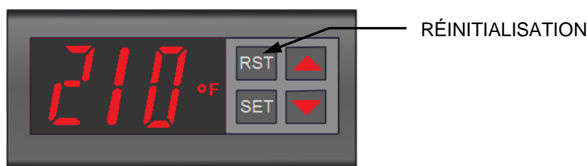
Figure 5-10 : Commutateur de limite de surchauffe à réinitialisation manuelle
