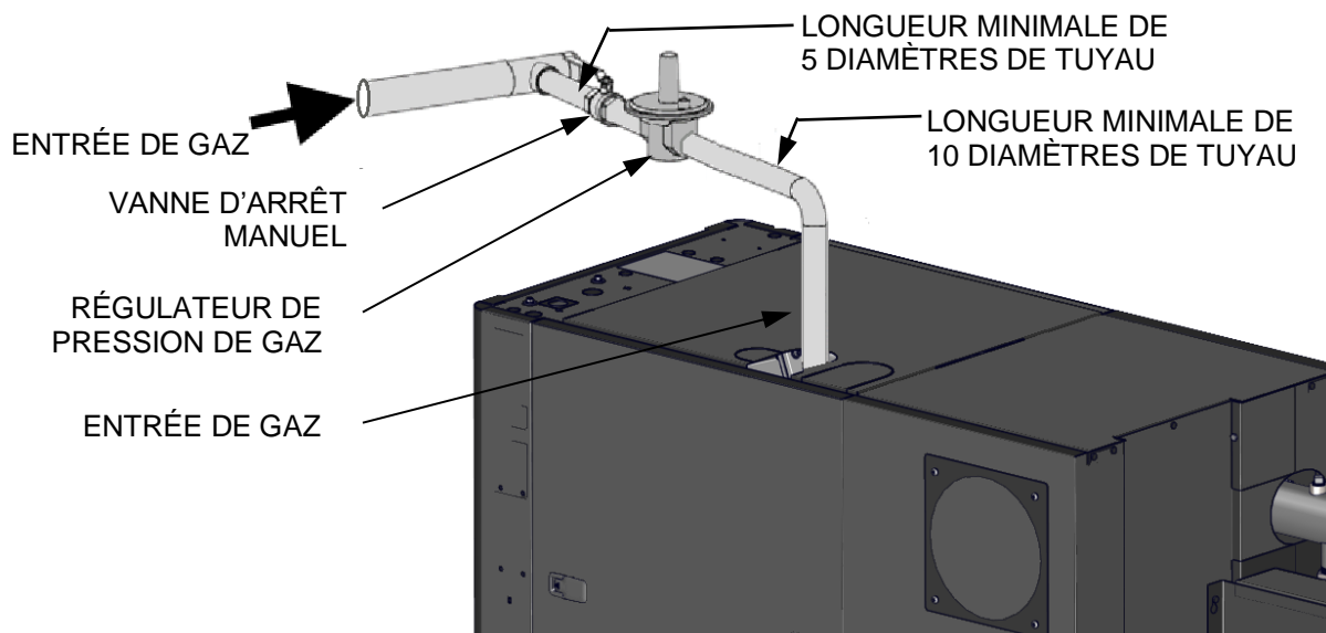
Figure 2-11 : Régulateur de gaz et vanne d'arrêt manuel
