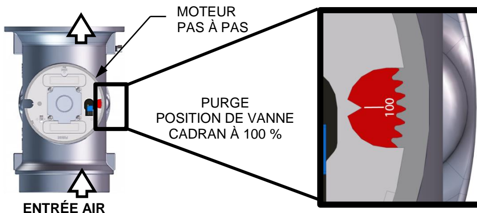
Figure 4-2 : Vanne air/carburant en position de purge
