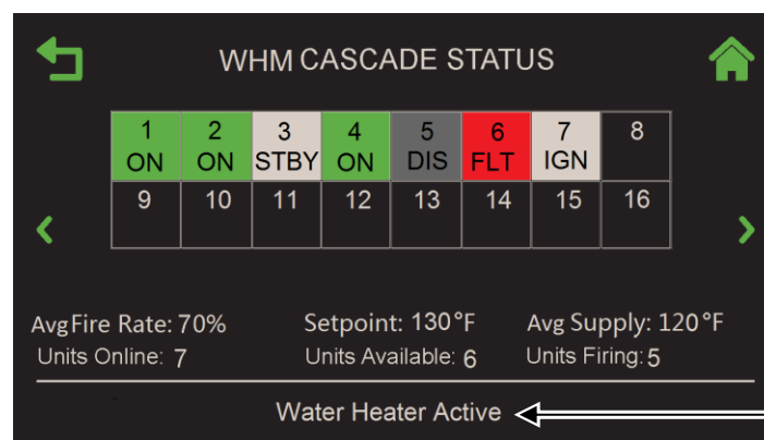
Figure 8-3 : Écran de la WHM Cascade Status
