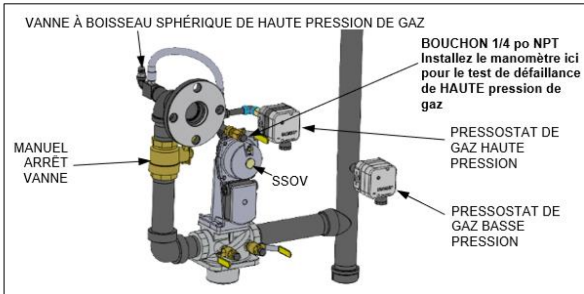
Figure 6-4 : Test de défaillance de HAUTE pression de gaz
