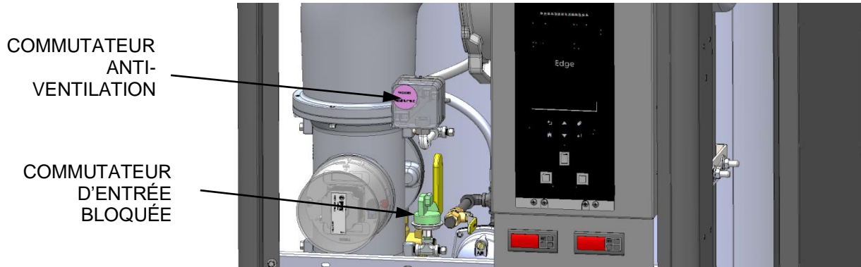
Figure 4-3 : Commutateur « Blocked Inlet » et « Blower Proof »
