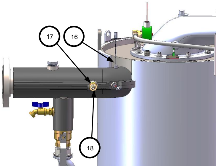
VUE ARRIÈRE GAUCHE DU DESSUS
