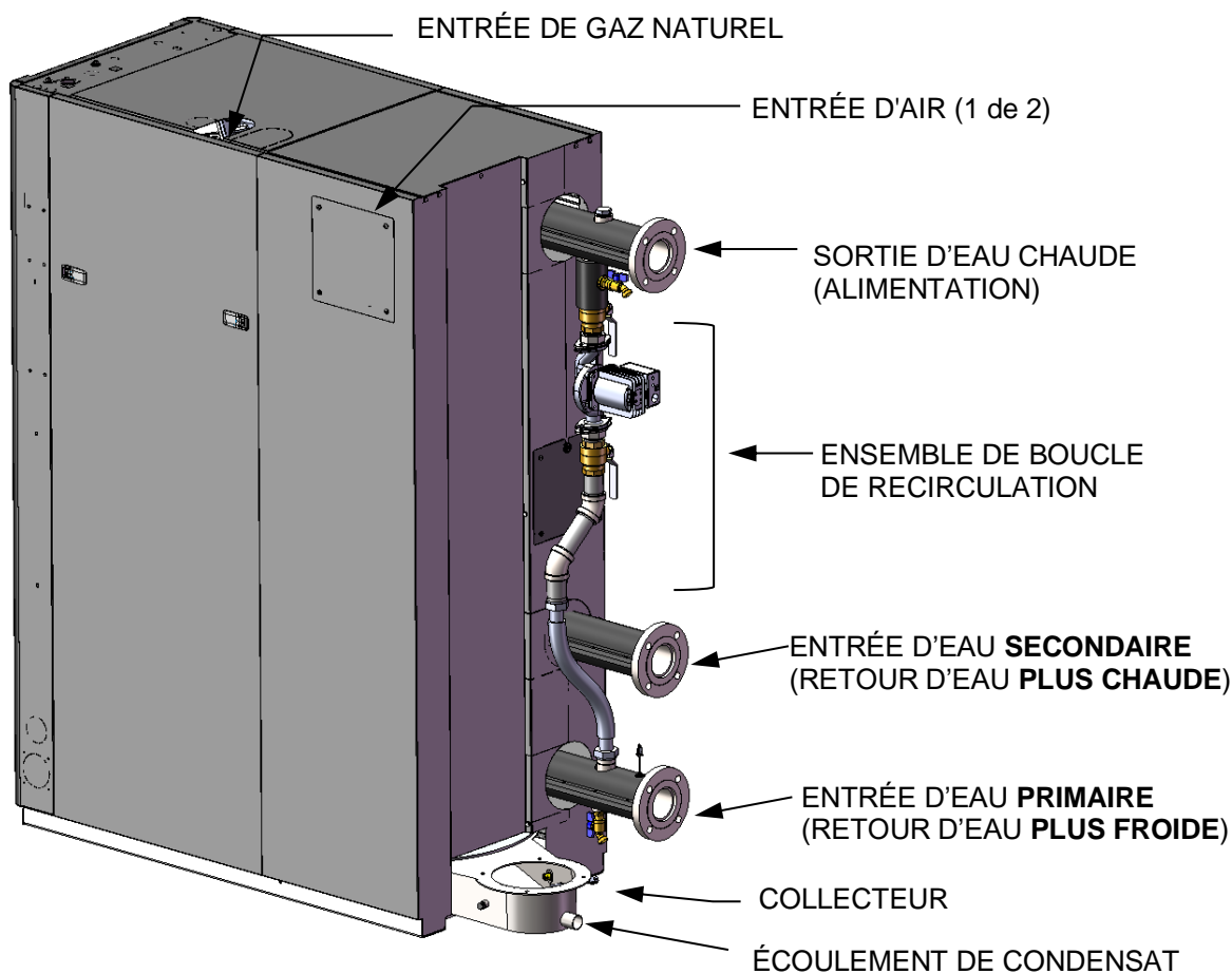
Figure 2-5 : Emplacements d'alimentation et de retour
