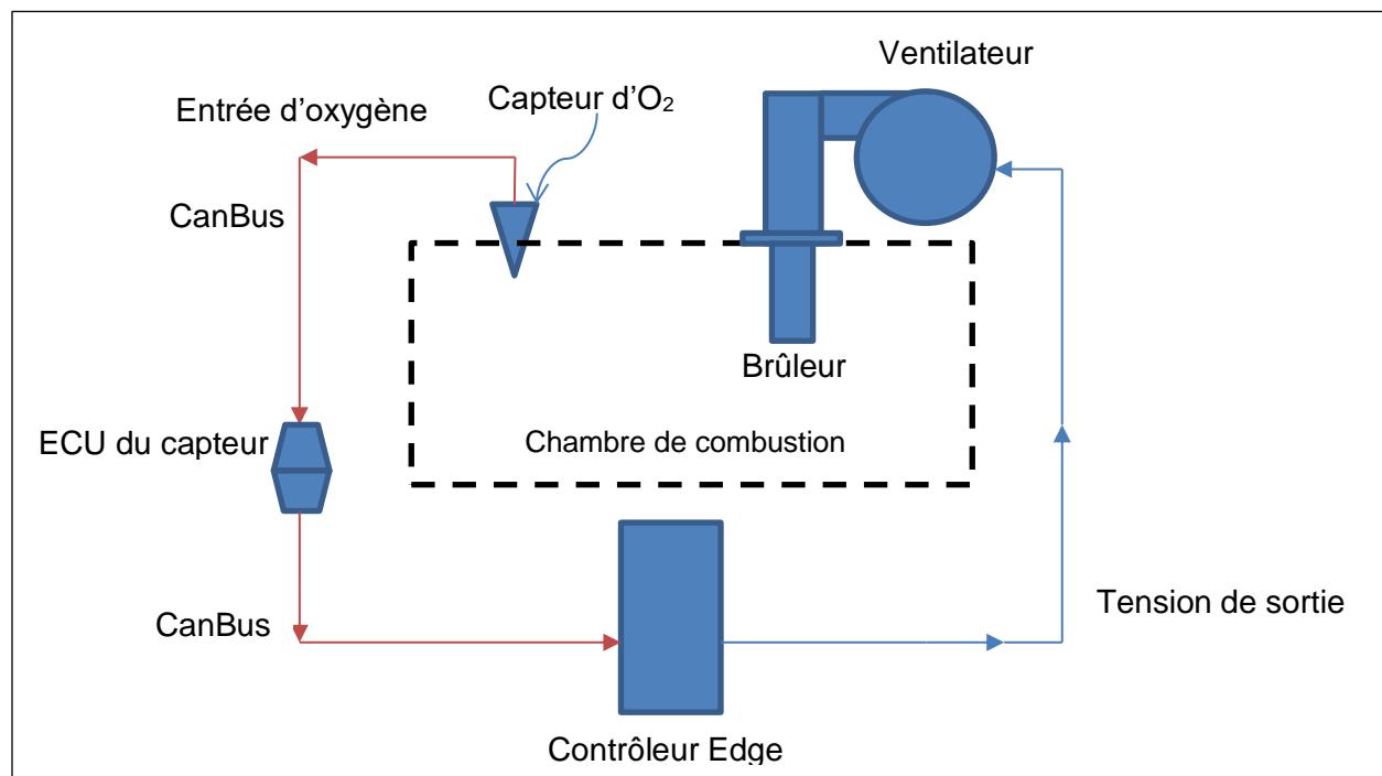
Figure 9-1 : Diagramme O 2 Trim simplifié
