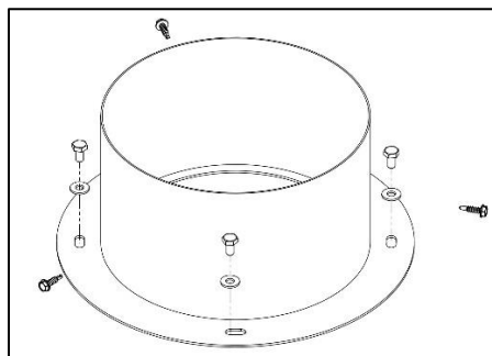
Figure 2-1: Serrez les trois vis à 120 degrés l'une de l'autre
