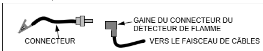
Figure 6-9 : Branchement du générateur de signal de flamme
