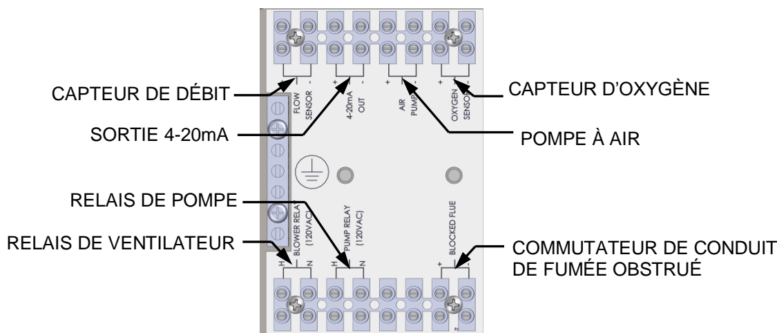
Figure 2-14 : Bornes du panneau d'alimentation secondaire
