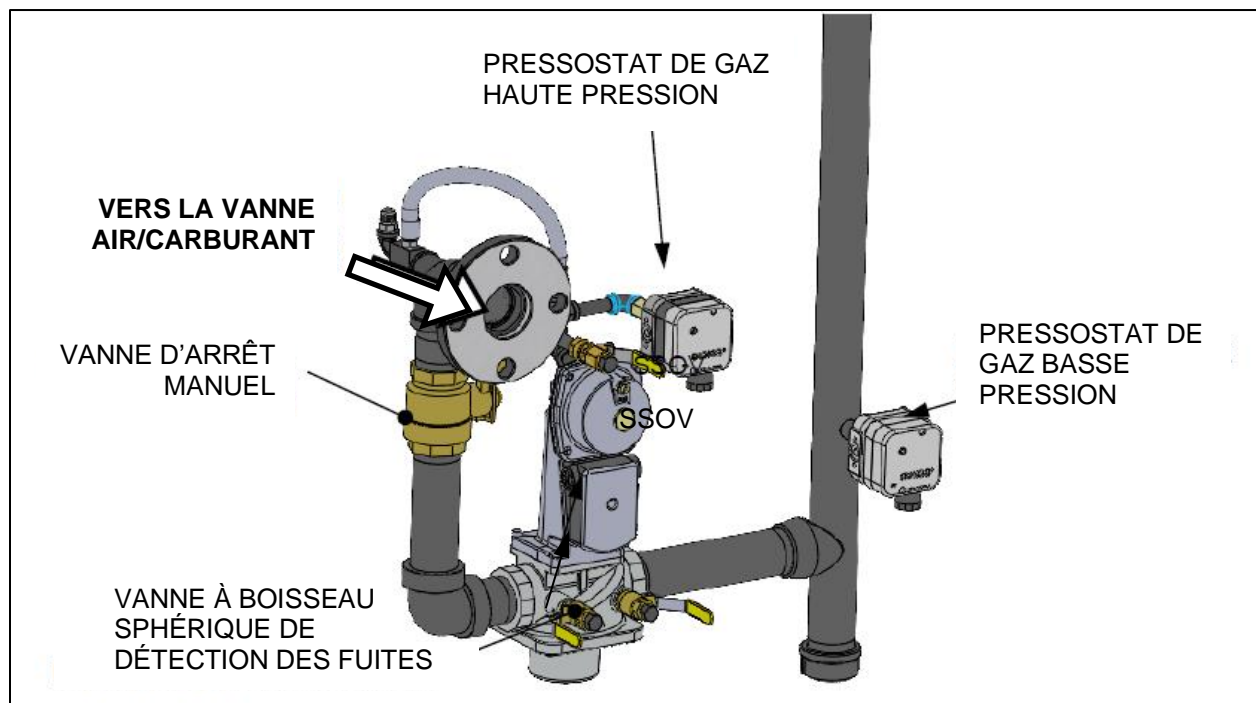
Figure 10-1 : Emplacement des composants du circuit de gaz (P/N 22362C illustré)
