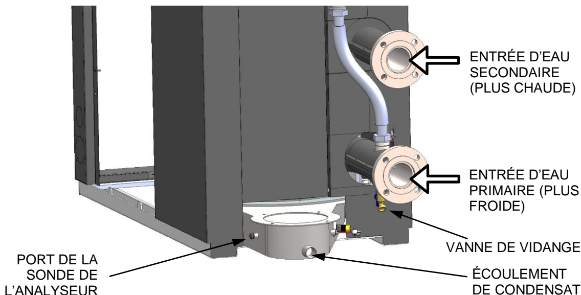
Figure 5-3 : Emplacement du port de la sonde de l'analyseur
