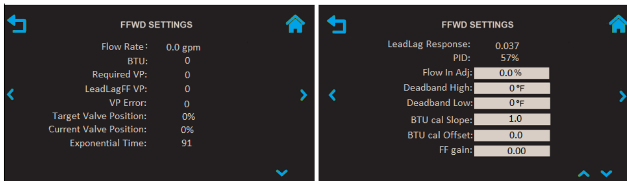
Figure 5-12 : Écrans de paramètres FFDW
