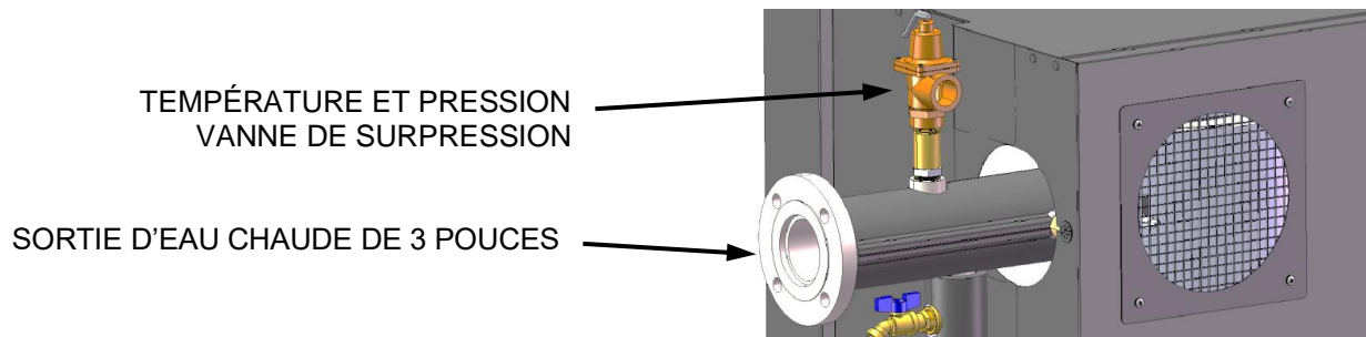
Figure 2.9 : Emplacement de la vanne de surpression P&T
