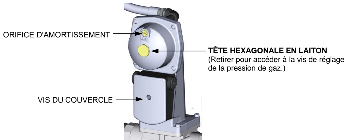
Figure 10-3 : Actionneur de la SSOV avec ajustement de la pression de gaz (SKP25)
