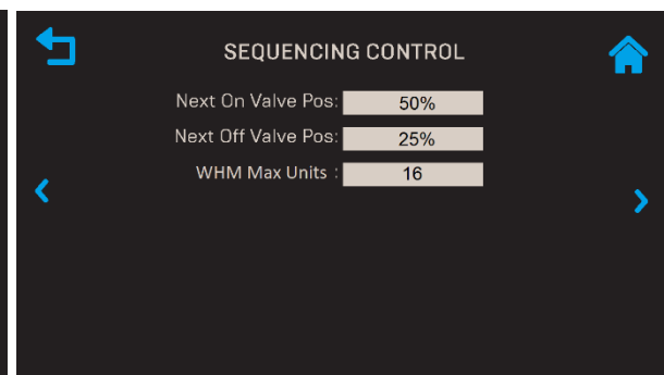
Écran du WHM Manager
