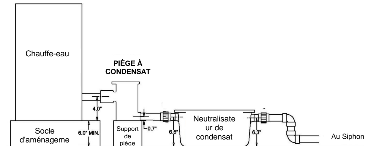
Figure 2-3 : Installation de cuve à neutralisateur de condensat
