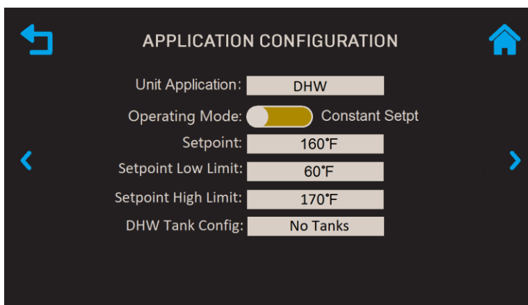
Figure 5-14 : Écran Configuration de l'application
