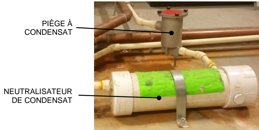
Figure 7-6 : Piège à condensat et neutralisateur
