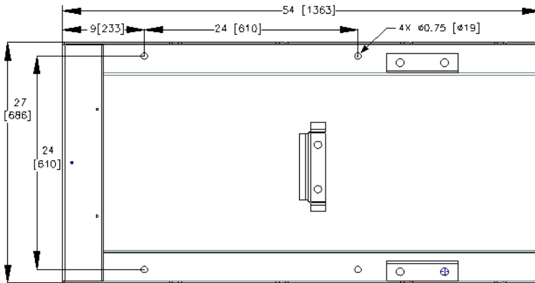
Figure 2-2 : Emplacement des boulons d'ancrage
