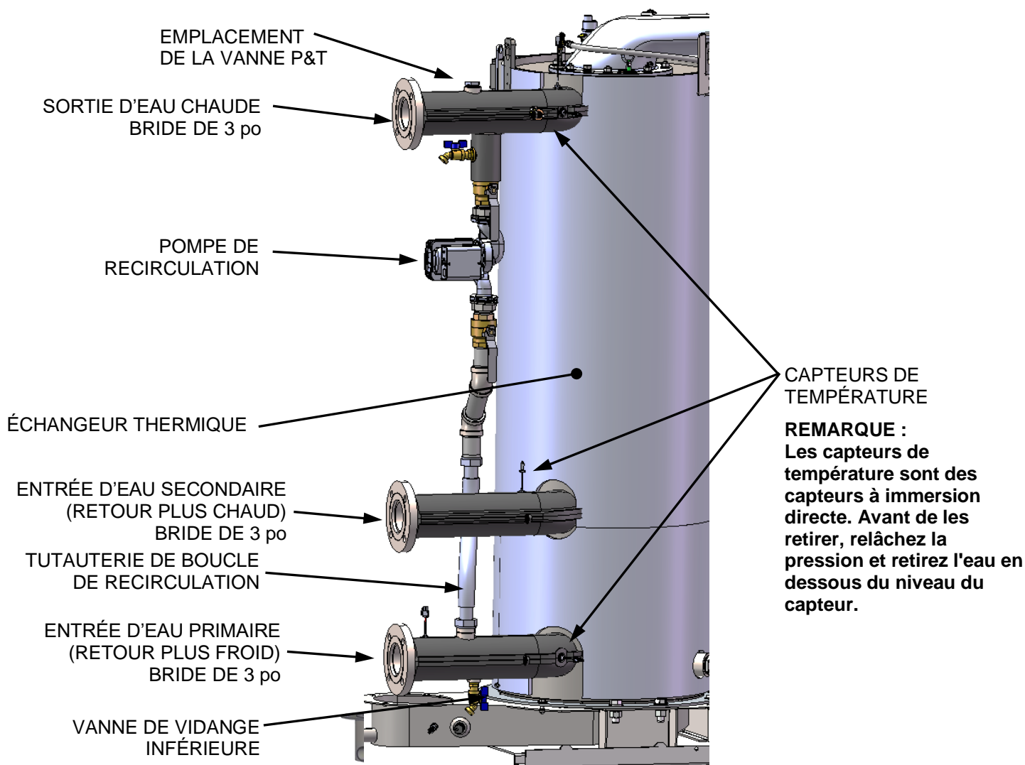
Figure 2-6 : Vue arrière de la boucle de recirculation – Panneaux arrière et évent d'échappement retirés
