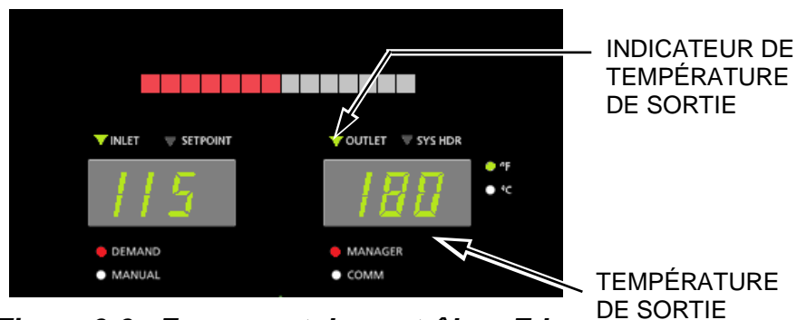
Figure 6-6 : Face avant du contrôleur Edge
