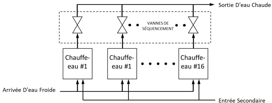
Figure 8-1 : Schéma fonctionnel simplifié - WHM (Water Heater Management)
