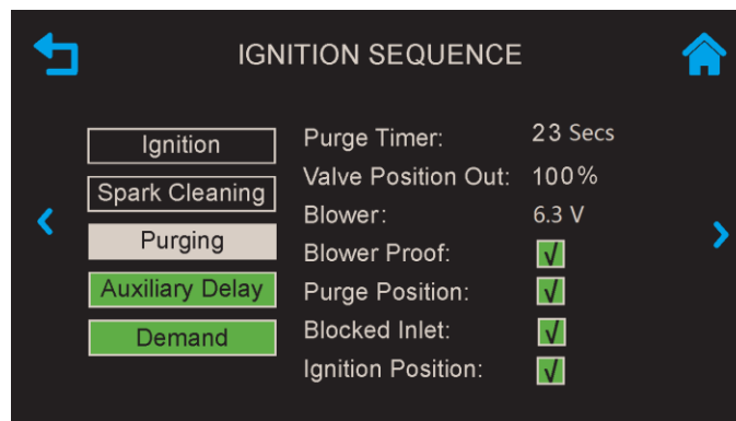
Figure 4-4 : Écran Séquence d'allumage — Purging
