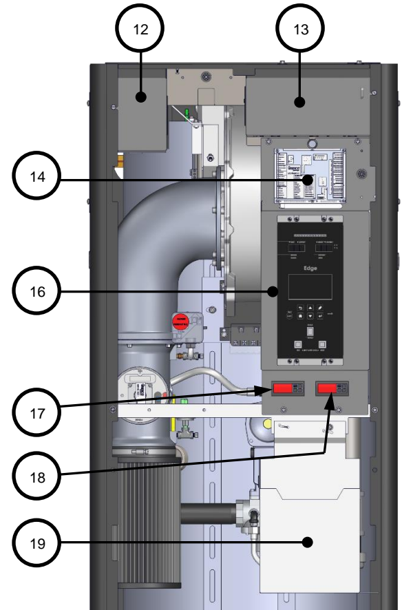
VUE AVANT PARTIELLE PANNEAU AVANT DÉMONTÉ
