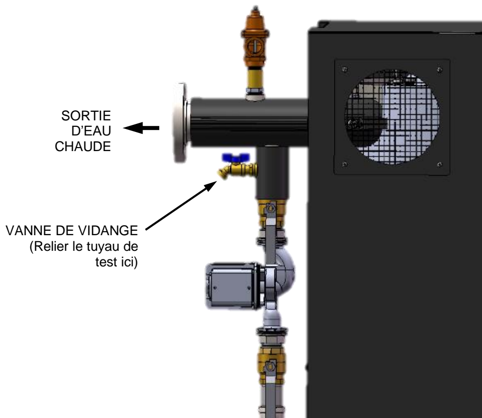
Figure 2-7 : Emplacement du tuyau de test
