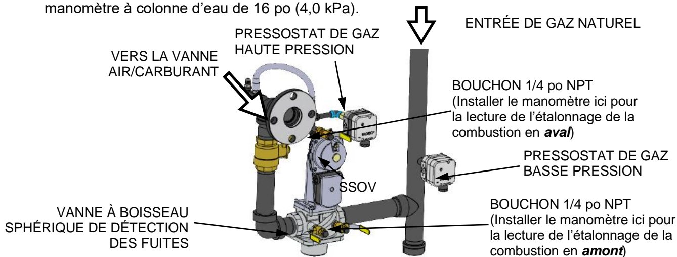
Figure 5-2 : Emplacement du bouchon de gaz de 1/4 po
