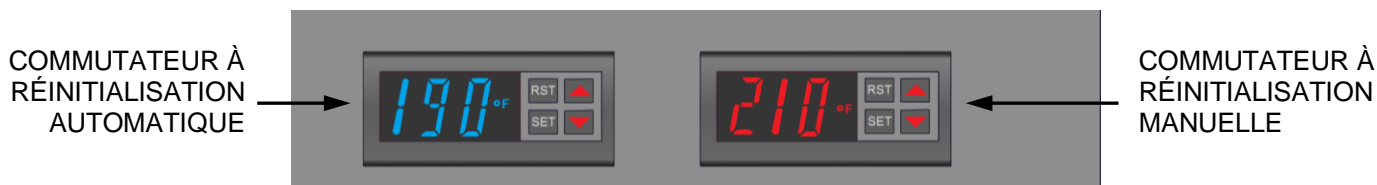
Figure 5-8 : Commutateurs de limite de surchauffe
