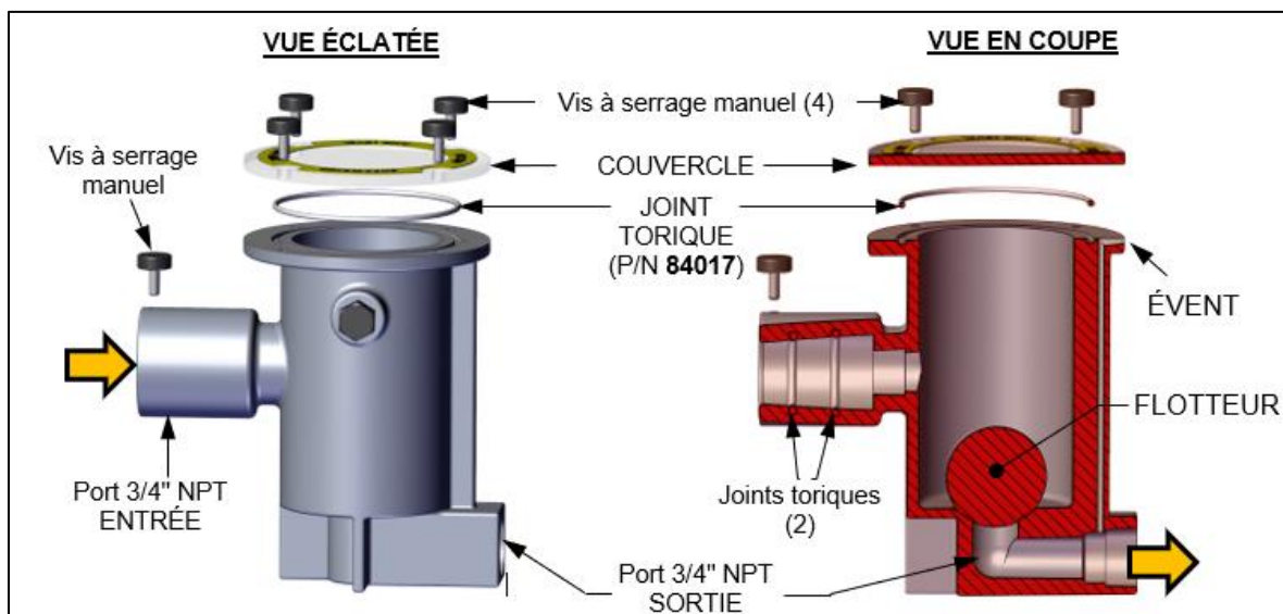
Figure 7-5 : Piège à condensat extérieur - Vue en coupe et vue éclatée
