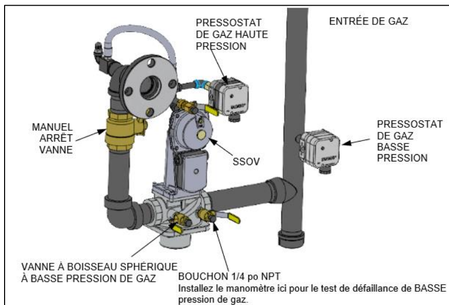
Figure 6-2 : Composants de test de BASSE pression de gaz
