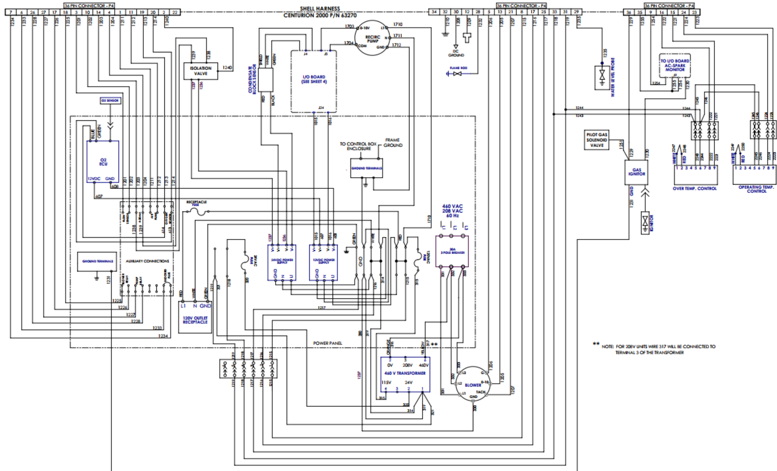
Centurion 2000 – Numéro de schéma : 68106 rév. C Fiche 1 sur 4
