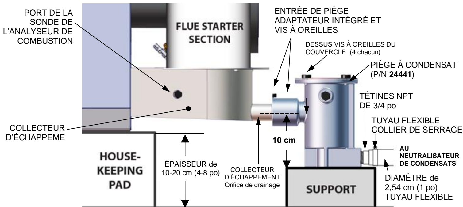
Figure 2-10 : Exemple d'installation de piège à condensat
