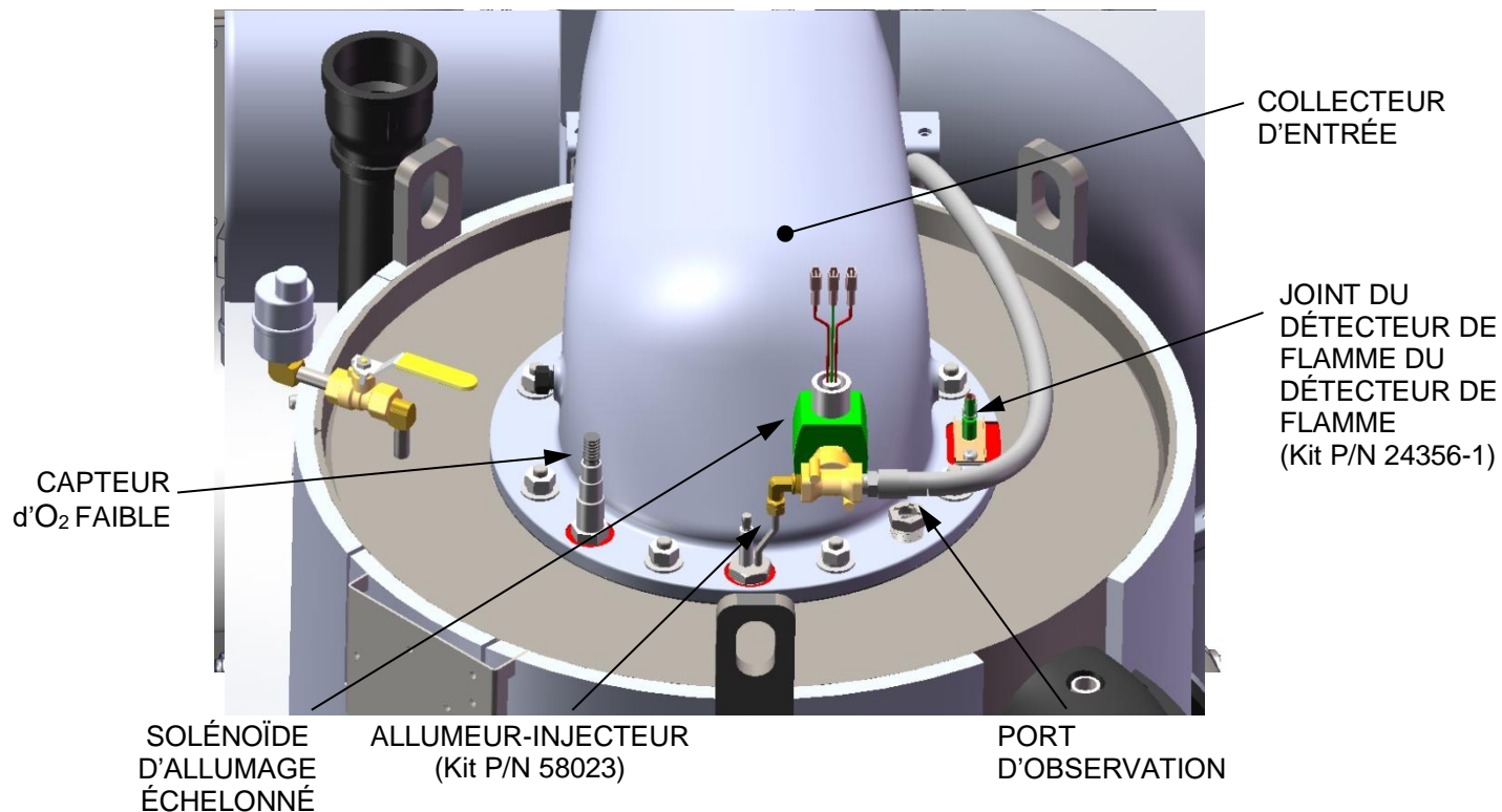
Figure 10-2 : Collecteur d'entrée et composants
