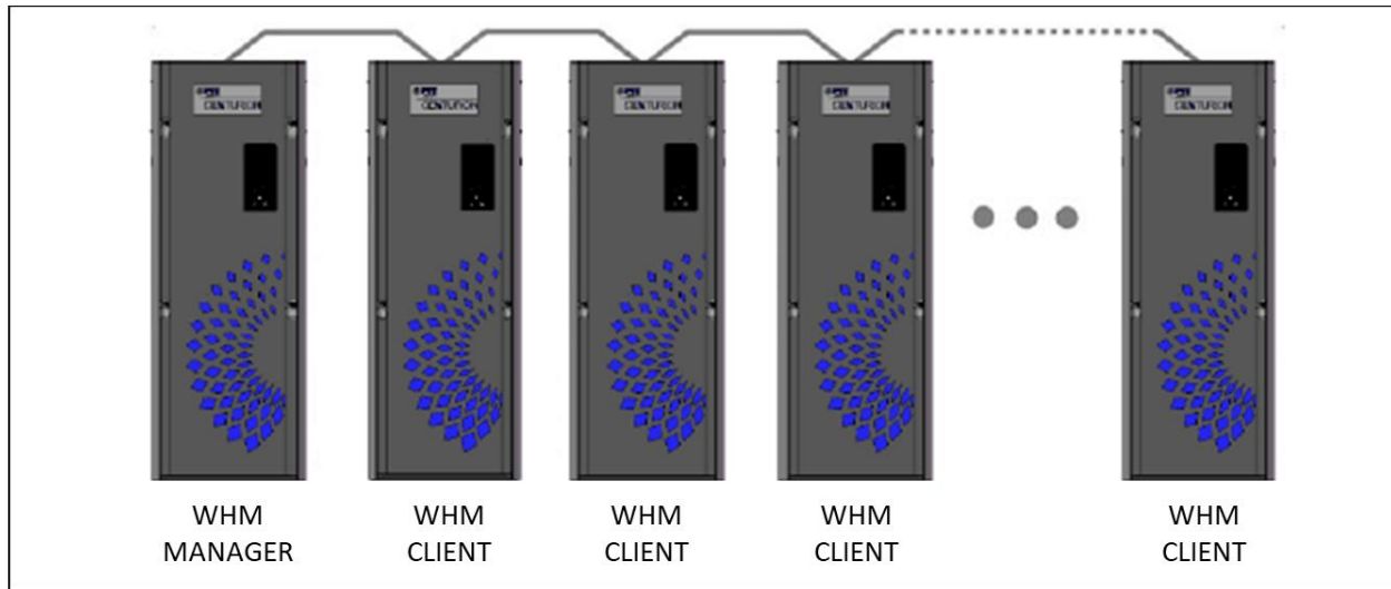
Figure 8-11 : Réseau Modbus/RS485 en chaîne classique
