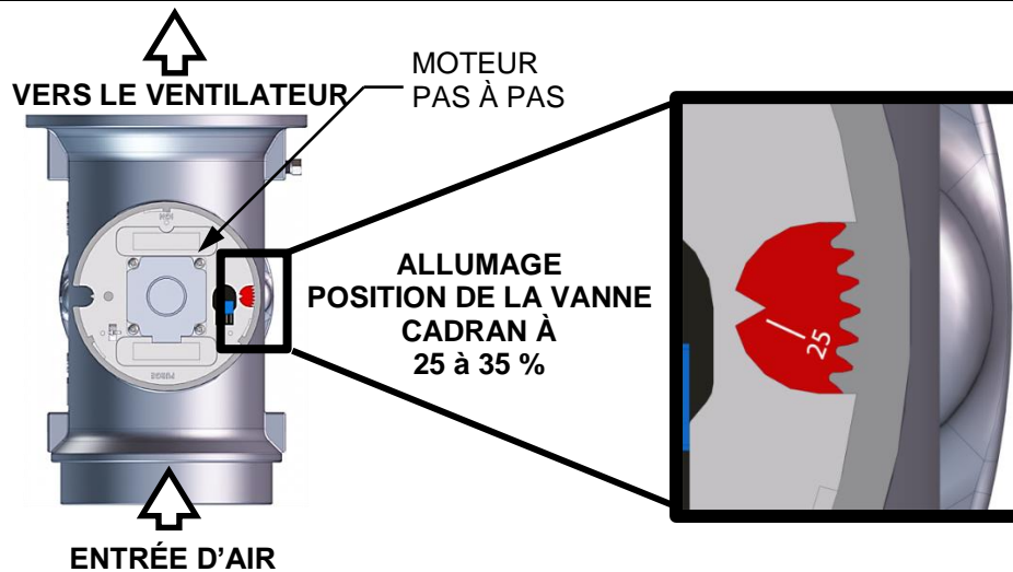
Figure 4-5 : Vanne air/carburant en position d'allumage
