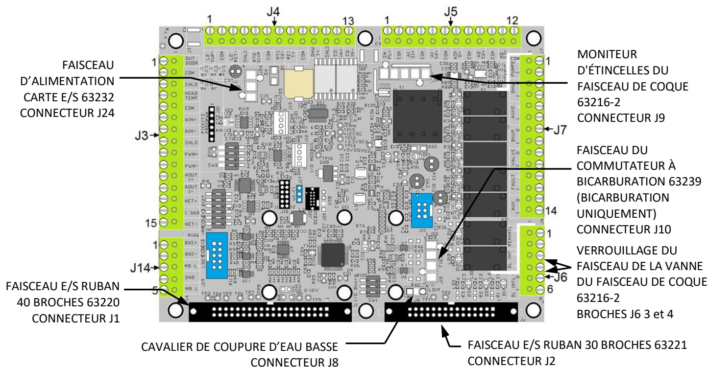
Figure 2-15 : Connexions des câbles de la carte E/S
