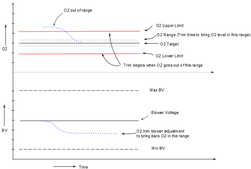
Figure 9-2 : Logique d'O 2 Trim
