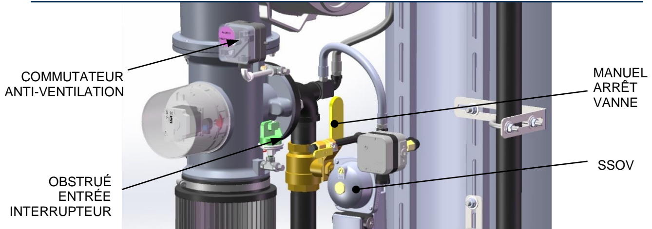
Figure 6-7 : Emplacement du commutateur d'entrée bloquée et du commutateur anti-ventilation
