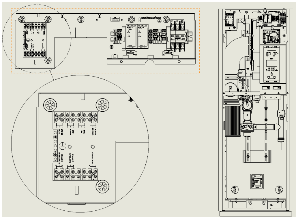
Figure 2-19 : Relais de la pompe du chauffe-eau
