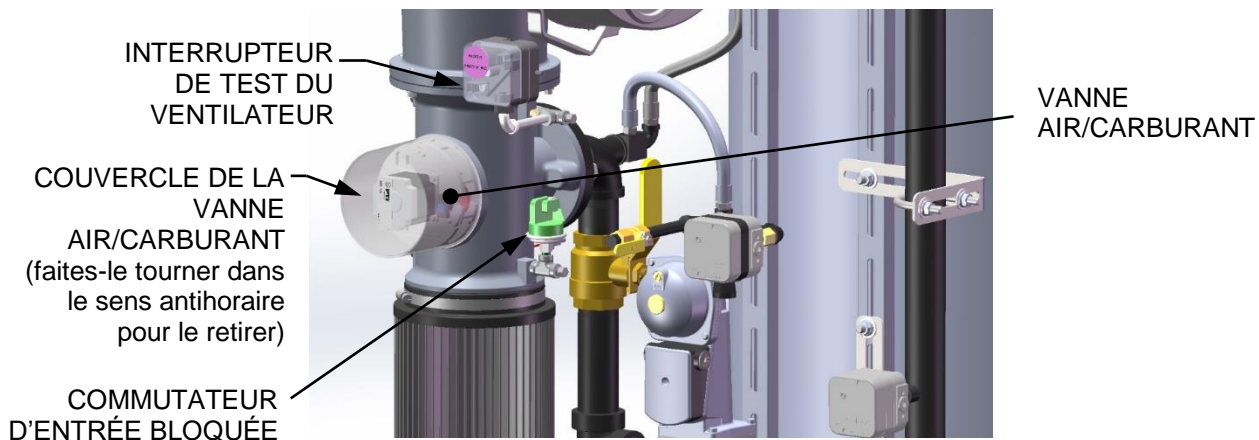
Figure 6-10 : Emplacement du couvercle de la vanne air/carburant
