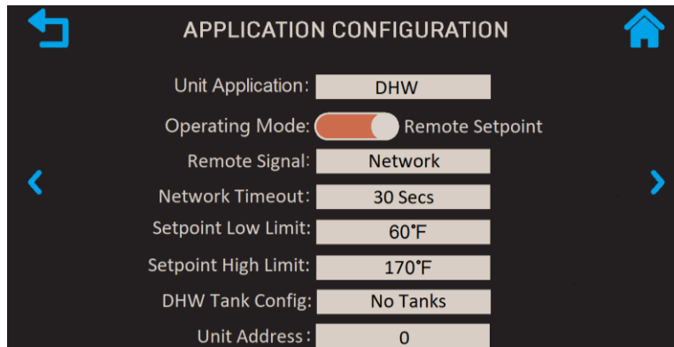
Figure 5-15 : Écran Configuration de l'application
