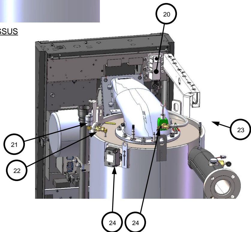
VUE SUPÉRIEURE ARRIÈRE
