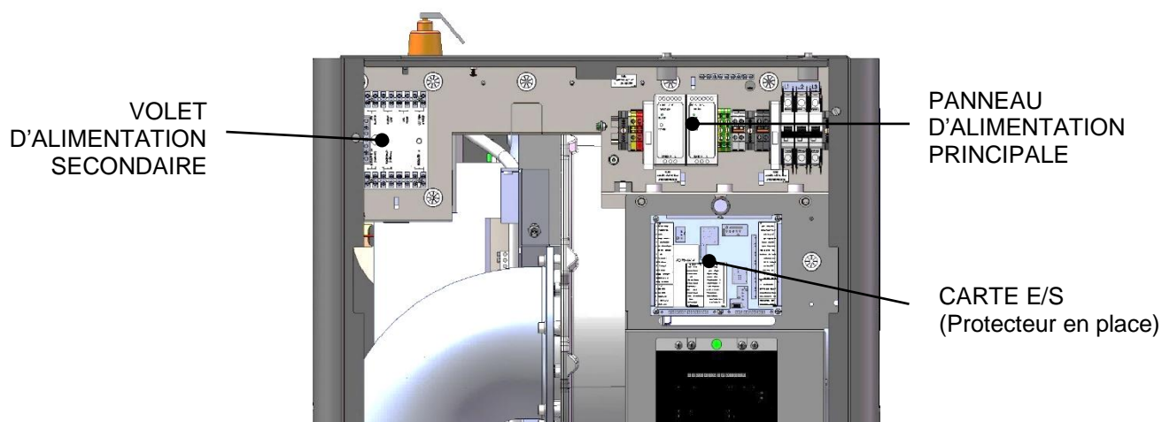
Figure 2-12 : Panneau d'alimentation
