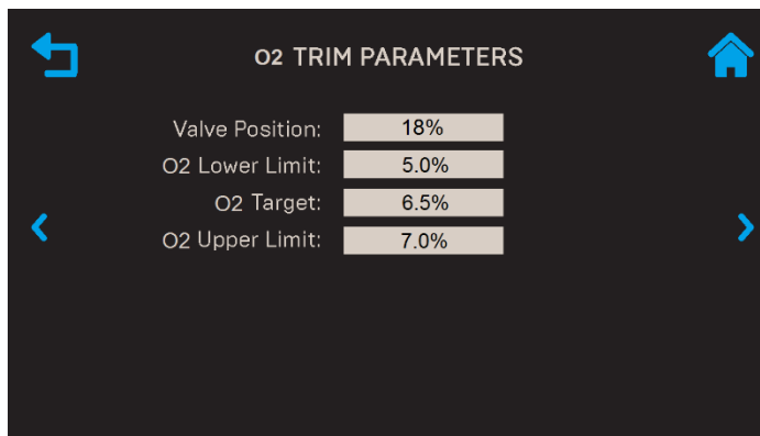
Figure 9-4 : Écran Paramètres de calage d'O 2
