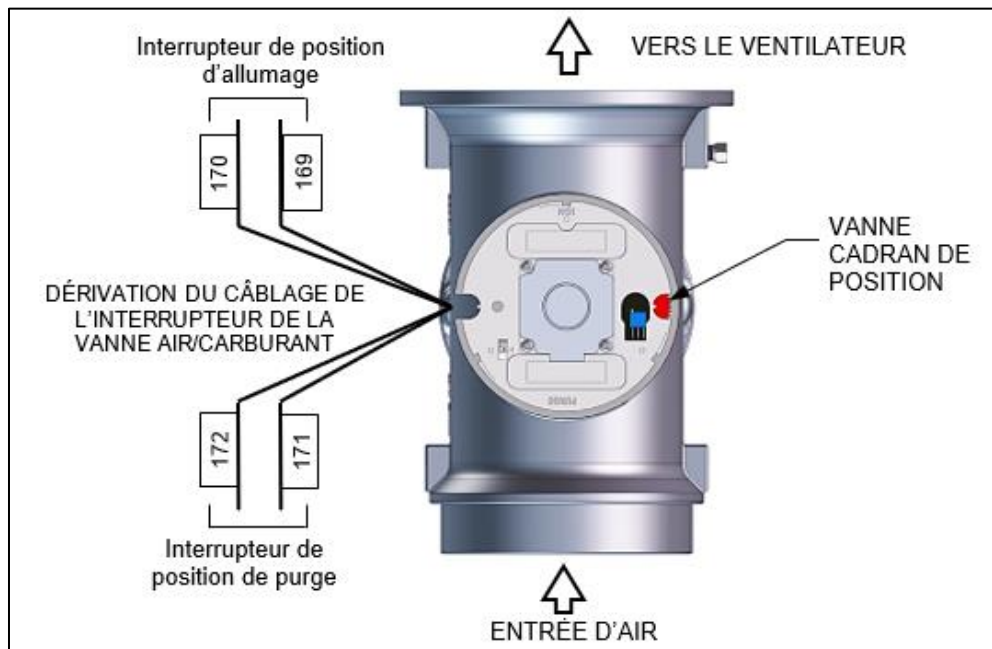
Figure 6-11 : Emplacement de la purge d'air/carburant et de l'allumage
