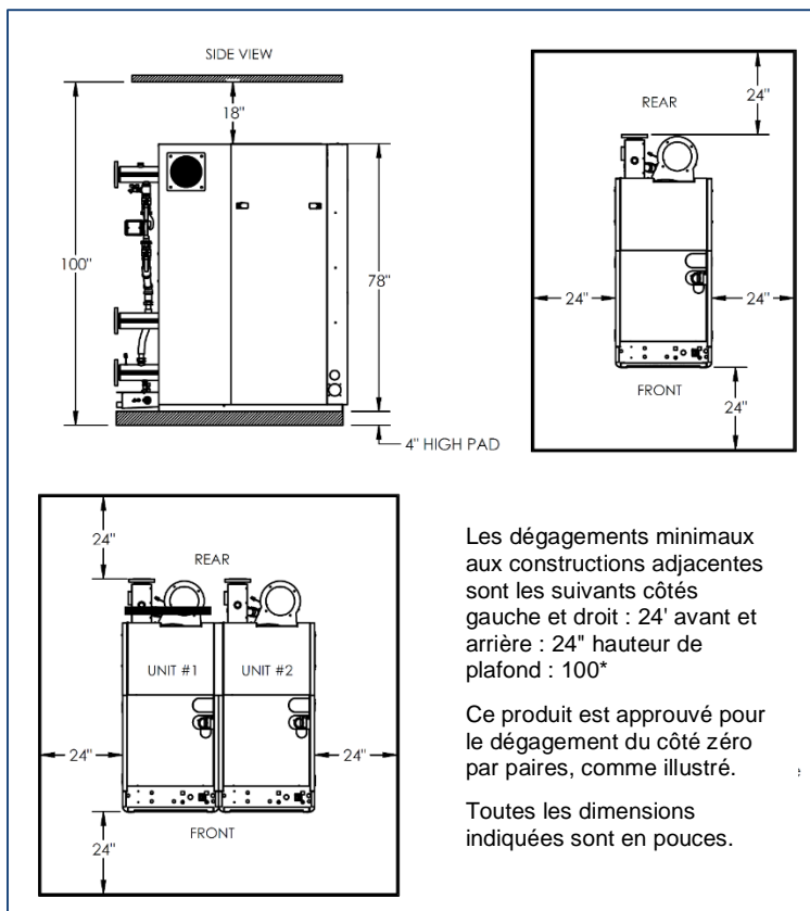
Figure 2-1 : Dégagements
