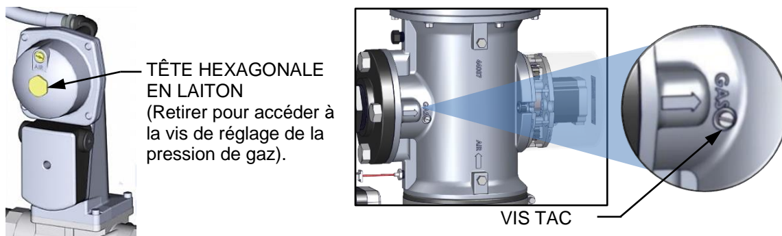
Figure 5-4 : Emplacement de la vis de réglage de la pression du gaz et de la vis TAC
