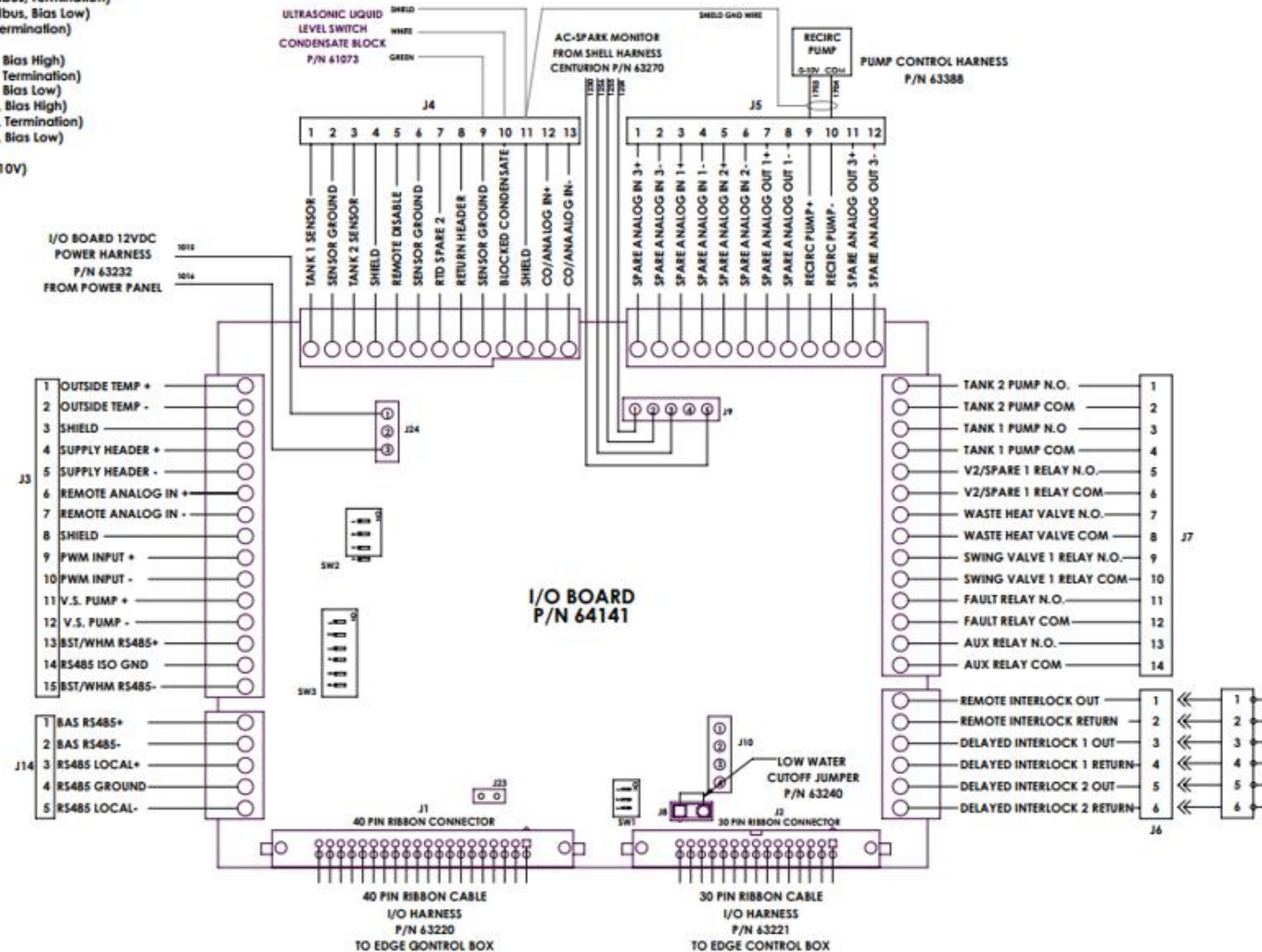
Centurion 2000 – Numéro de schéma : 68106 rév. C Fiche 4 sur 4
