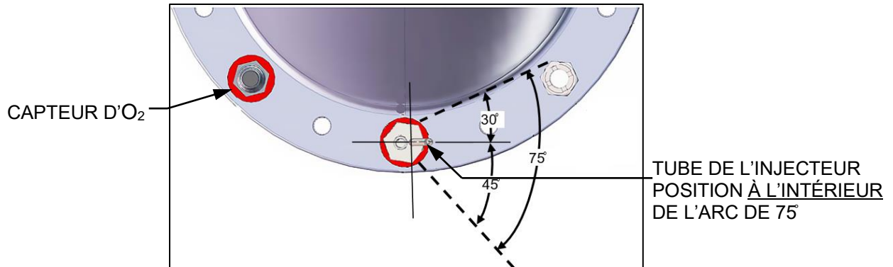
Figure 7-2. Orientation de l'allumeur-injecteur
