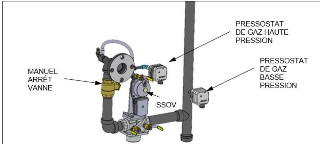
Figure 4-1 : Emplacement du SSOV
