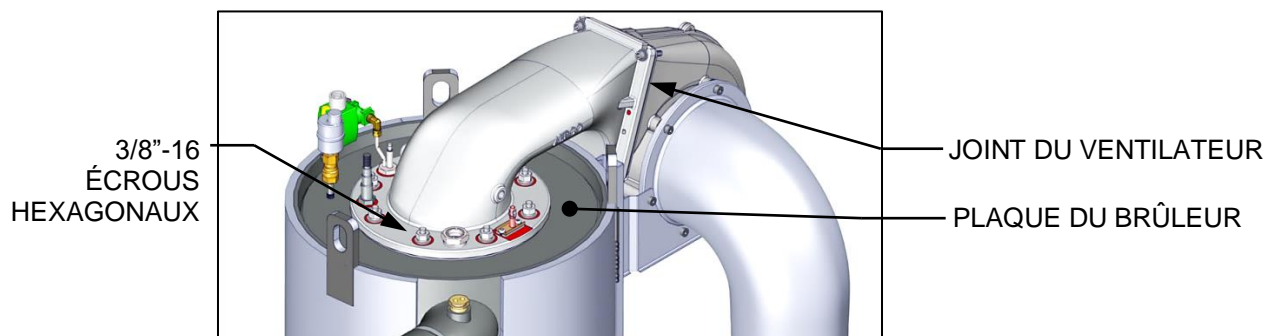
Figure 7-4 : Détails de montage de l'ensemble de brûleur
