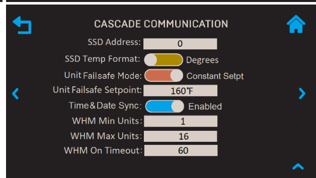
Écran Du WHM Manager
