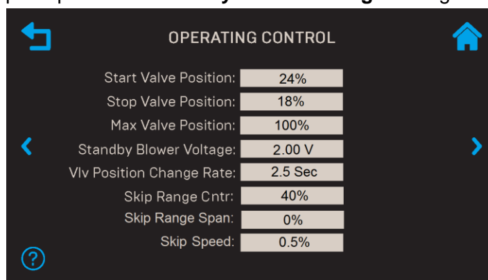
Figure 5-1 : Écran de Operating Control
