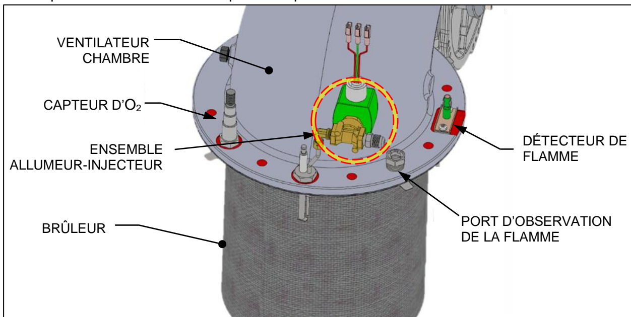
Figure 7-1 : Allumeur-injecteur et détecteur de flamme
